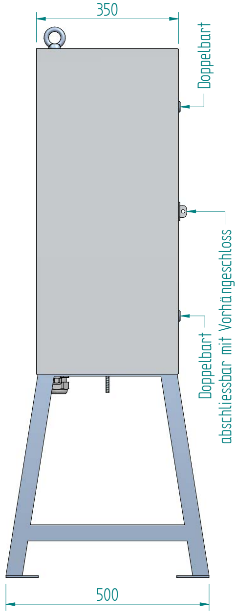
Schema Art.Nr. 231129
